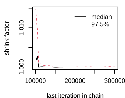
d.Erlotinib.Erlotinib_Autophagy
