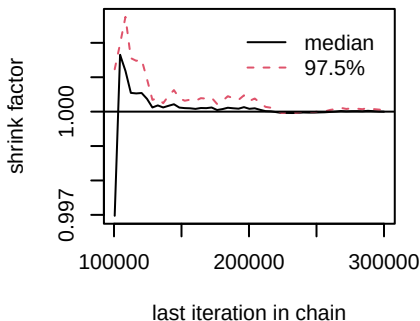
d.Erlotinib.Gefitinib_ERi
