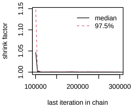
d.Erlotinib.DHFRi
