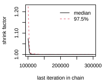
d.Osimertinib.Osimertinib_PD_L:
