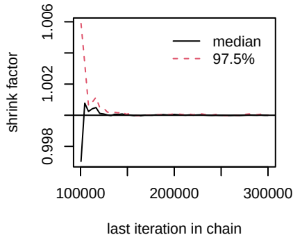
d.Erlotinib.Erlotinib_METi
