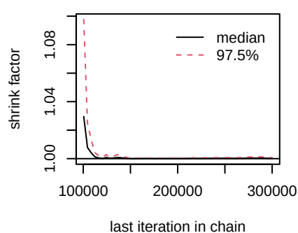
sd.d
