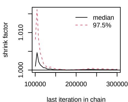
d.Erlotinib.Erlotinib_antiangio
